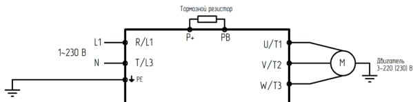
Рис. 3.2б. Подключение силовых клемм
