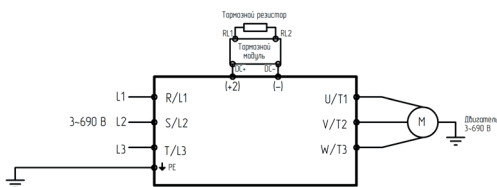
Рис. 3.2д. Подключение силовых клемм
