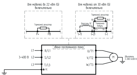
Рис. 3.2г. Подключение силовых клемм
